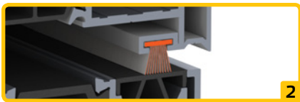
ZUSÄTZLICHE BÜRSTENDICHTUNG ALS NACHDICHTUNG
